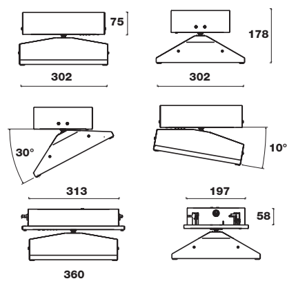
Mått (mm):
